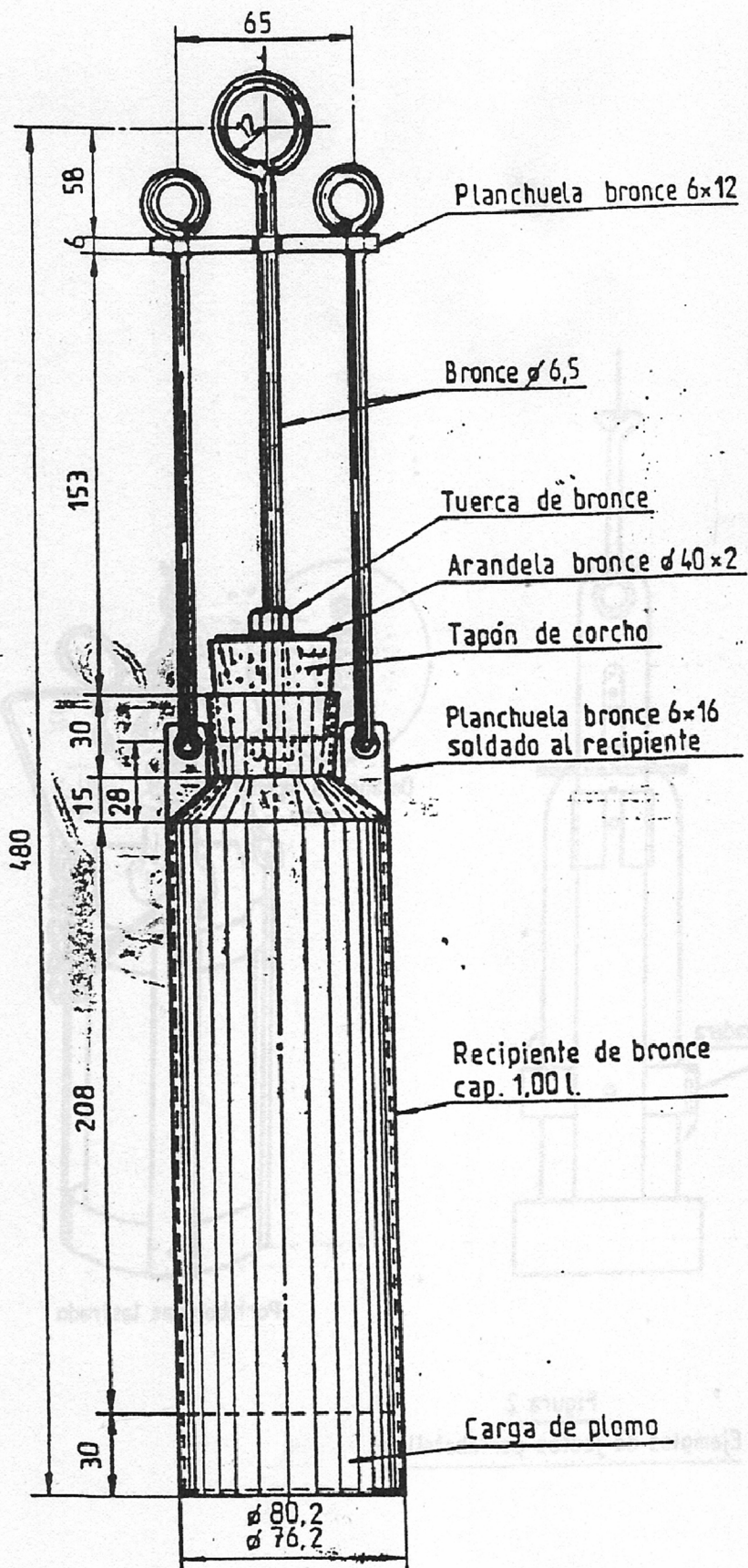
Figura 3 Dispositivo para extracción de muestras
