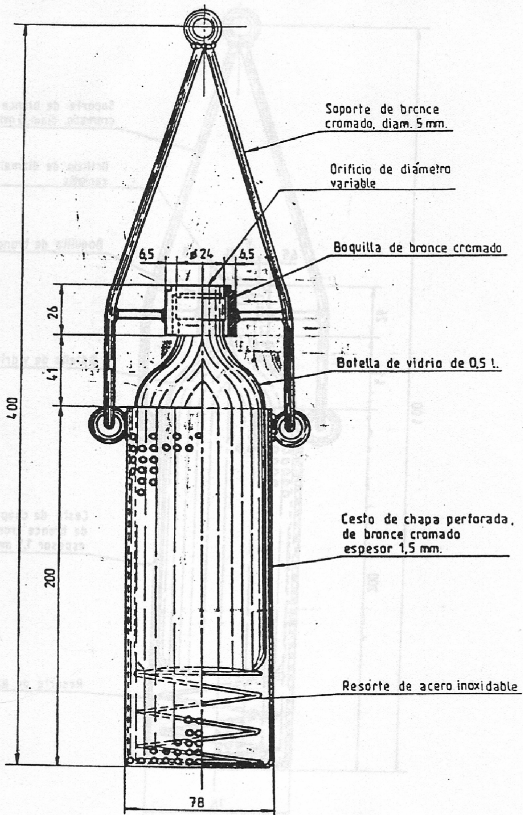
Figura 3 bis Sacamuestra para productos livianos
