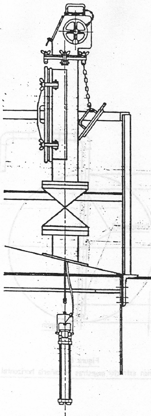
Figura 7 Dispositivo de cierre con trampa de vapor
