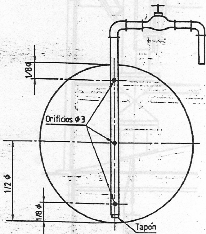
Figura 8 Conexión extractor muestras en cañería horizontal
