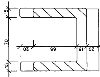
SECCION B-B ESC. 1:25
