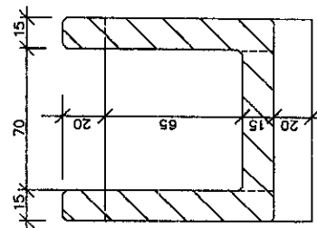
SECCION C-C ESC. 1:25
