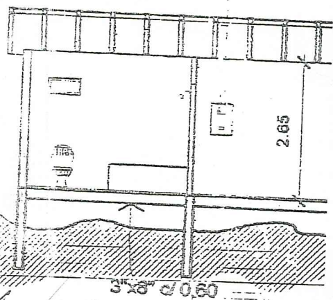
CORTE B-B (CABAÑAS)
