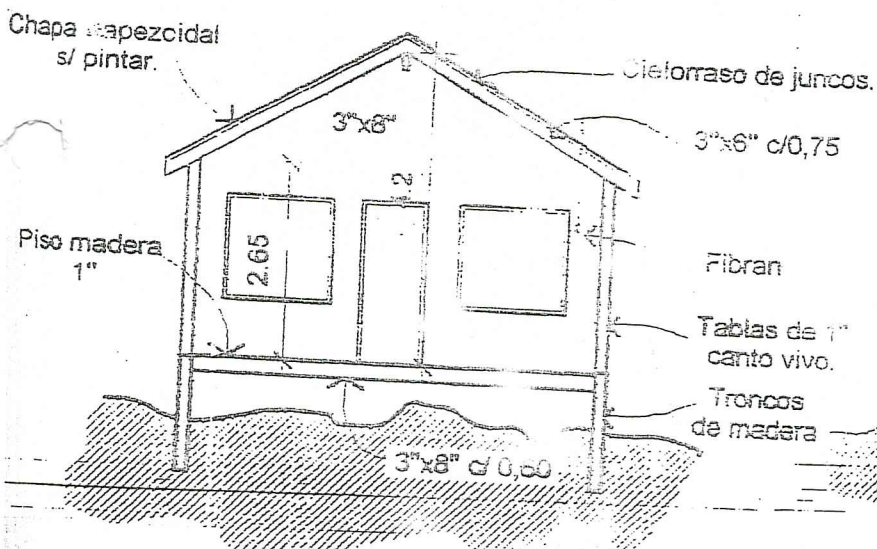
CORTE A-A (CABAÑAS)
