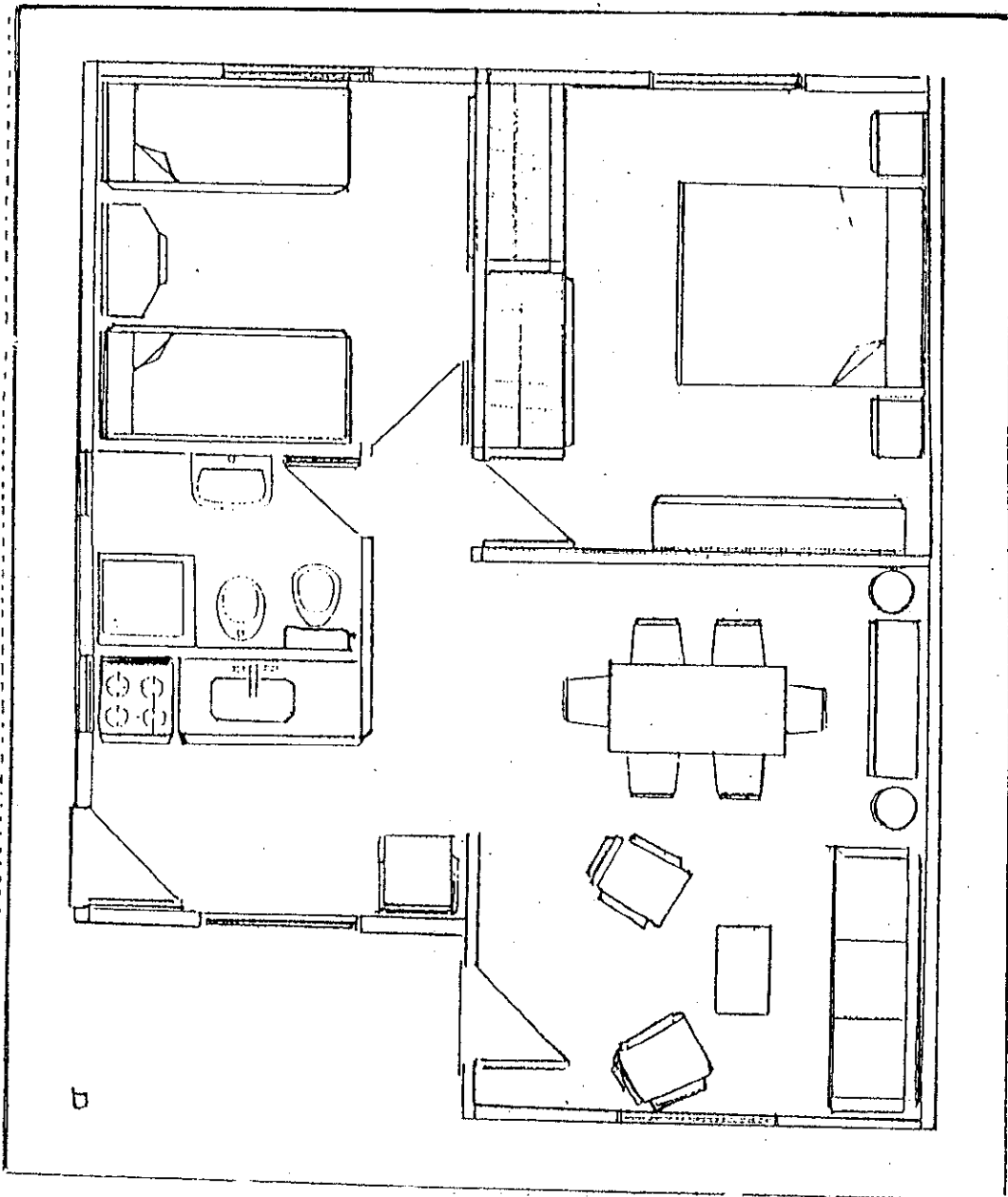
PROTOTIPO 2 Vivienda 2 dormitorios
